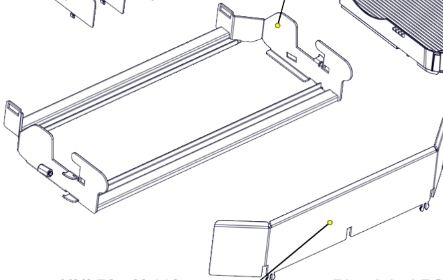
Frontstopper UNI 70 - H 113 mm Art. No 0070-00113
